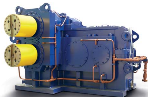
Горизонтальный редуктор с параллельными вальцами прокатного стана
