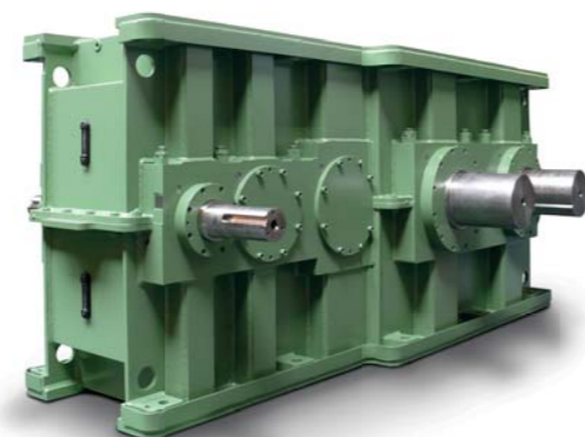
Симметричный редуктор для смесителя 520 л
