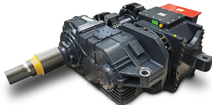
Kompletní pohon elektrické jednotky
