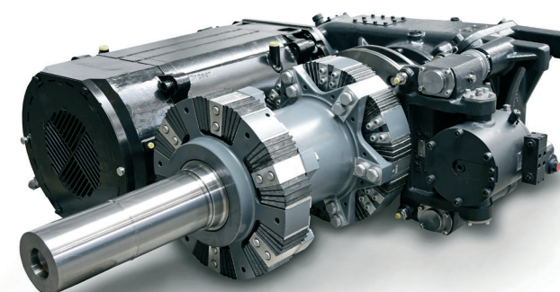
Kompletní pohon částečně nízkopodlažní tramvaje
