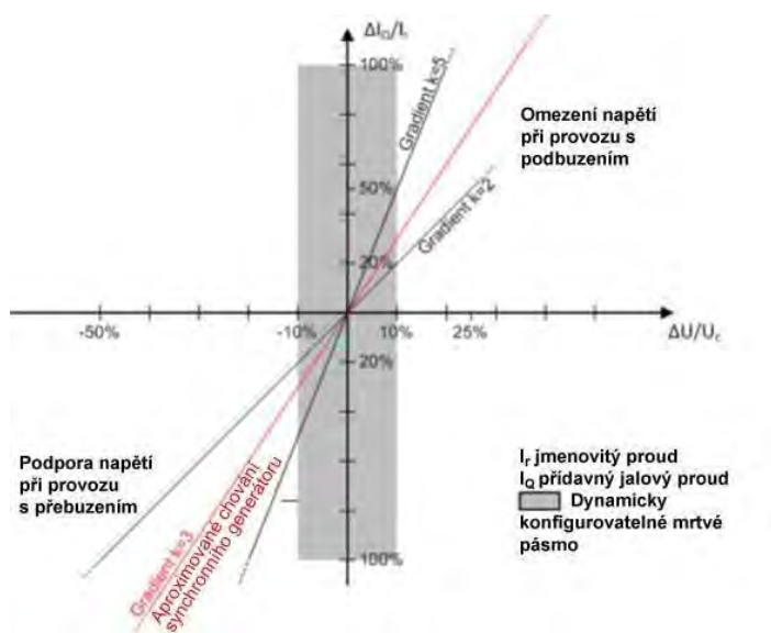
Obr. 4 Princip podpory napětí sítě při poruchách
