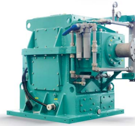
Редуктор для противопожарного насоса
