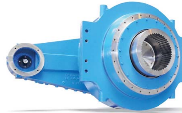
Редуктор для самоподъёмной системы нефтяных платформ
