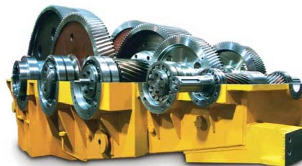
Редуктор подъема и выдвижения стрелы колеса
