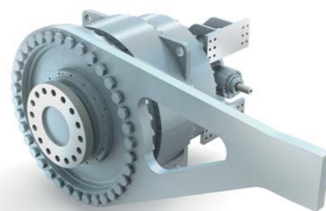
Коническо-планетарный редуктор Orbi-fleX колесных и гусеничных осей
