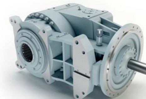
AFC převodovka hřeblového dopravníku
