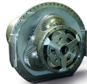
Planetová převodovka těžkých důlních vozidel
