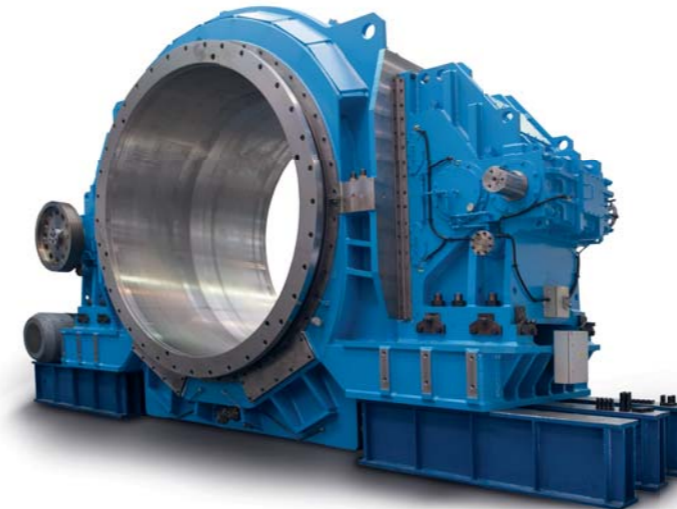
Привод горизонтальной шаровой мельницы с двумя редукторами типа SD мощностью 2.0 МВт
