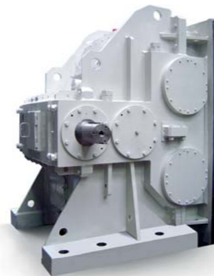
Редуктор серии / типа (2.2-3.3 МВт) для привода горизонтальной шаровой мельницы
