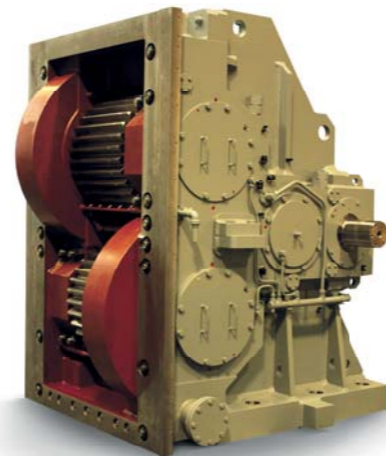
Редуктор серии / типа SD (4.1 – 6.0 МВт) для привода горизонтальной мельницы
