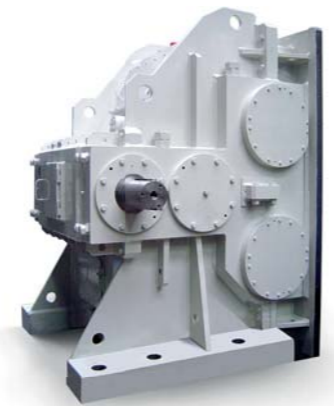
SD-Typ Getriebe für horizontale Kugelmühlen (2,5 - 3,3 MW)
