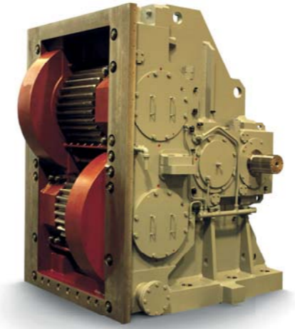
SD-Typ Getriebe für horizontale Kugelmühlen (4,1 - 6,0 MW)
