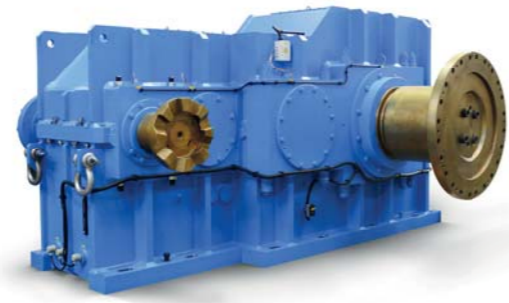
ZTE-Typ Getriebe für Rotationsöfen
