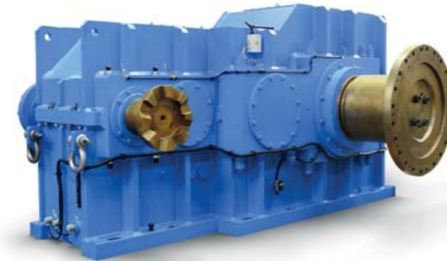
Převodovka typu ZTE pro rotační pec
