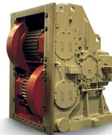
Převodovka typu SD (4.1 - 6.0 MW) pro pohon horizontálního mlýnu
